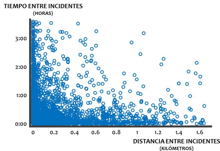
Figura 1. Esta gráfica muestra la distancia y la diferencia en tiempo de llamadas que sí están relacionadas entre sí. Cada punto representa una pareja de llamadas.
