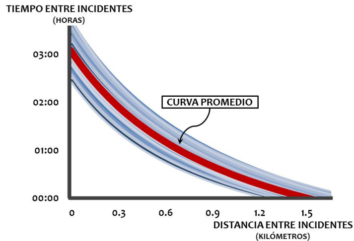
Figura 3. Representación de la curva definida por los puntos de corte para distintos soportes del ruido. Solo se ilustran las dimensiones de distancia y tiempo y el término cuadrático distancia \times tiempo. La región crítica para relacionar incidentes se encuentra debajo de la curva.
