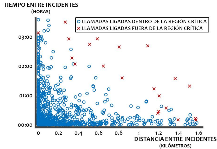
Figura 4. Clasificación de parejas relacionadas. Las 4 dimensiones finales del modelo están consideradas: distancia, tiempo, tipo y distancia \times tiempo. Los anillos son clasificados como relacionados y las \times representan los emparejamientos que el modelo deja fuera.
