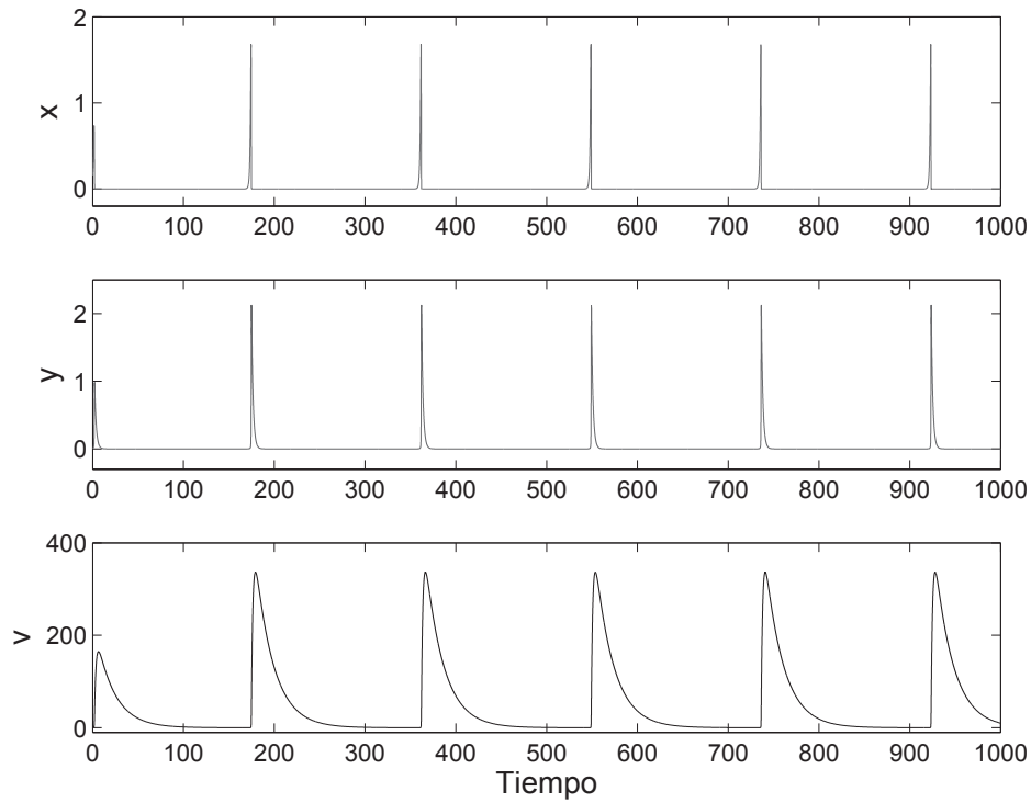
Figura 1: Periodicidad del sistema con un sólo tipo de infección, x representa organismos sanos, y organismos infectados y v representa los virus libres. Con los parámetros x = 0.15, y = 0.0010, v = 0.015, r = 1, m = 0.75, \beta = 0.5, \mu = 0.5, \delta = 0.05, k = 100, a = 0.75 y C = 0.08 .
